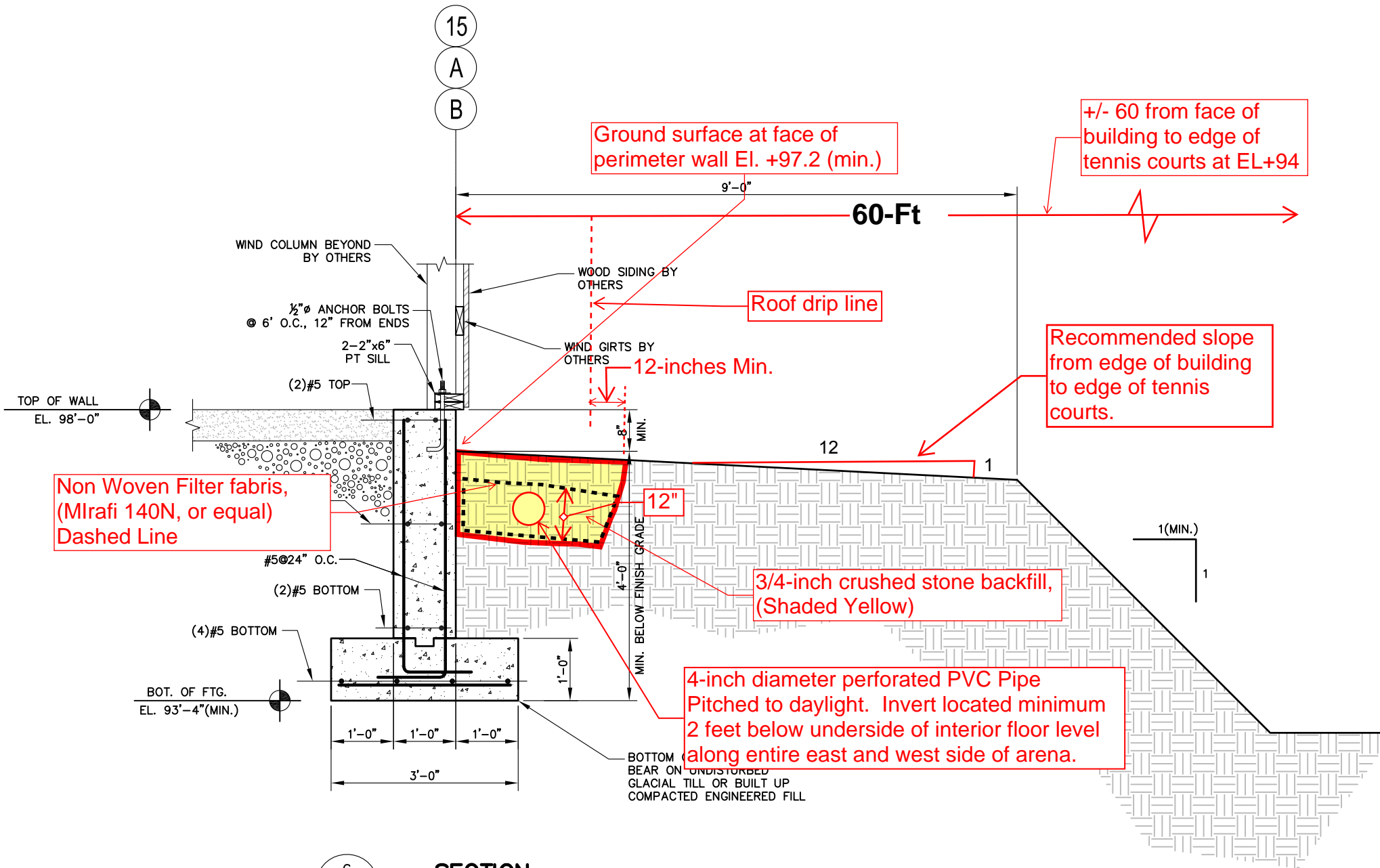
6 SECTION F1 SCALE: 3/4"=1'-0"
